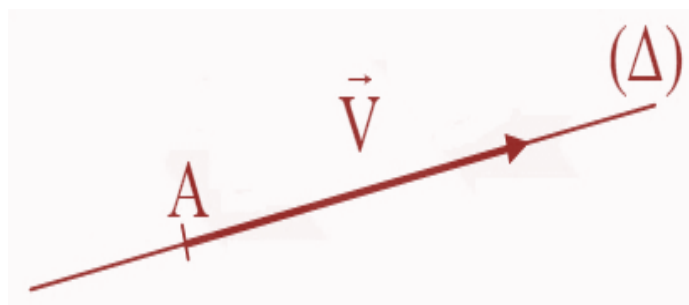
Figure. 2 : vecteur lié
