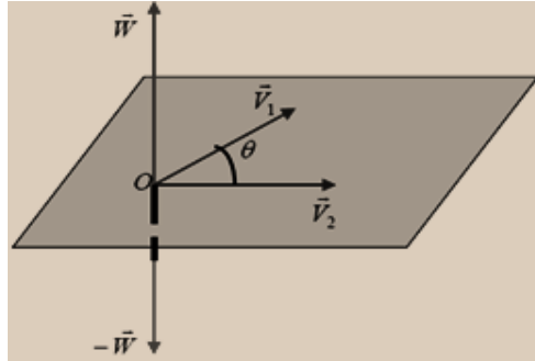
Figure. 11 : Produit vectoriel
