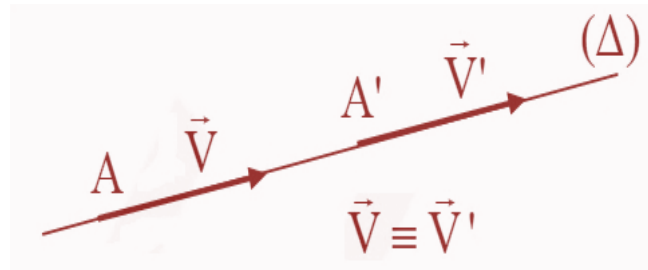
Figure. 3 : Vecteur glissant
