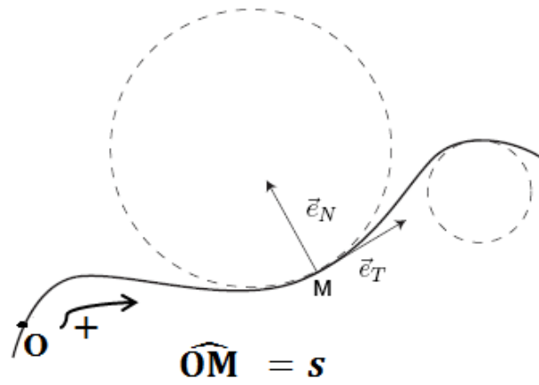
Figure. 27- Coordonnées curvilignes
