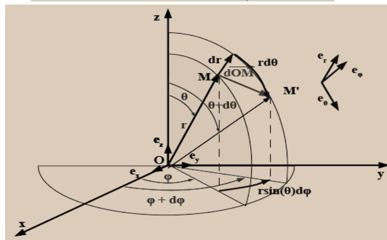
Figure 25 – Déplacement élémentaire en coordonnées sphériques
