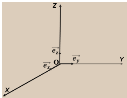
Fig. 15 : base orthonormée directe
