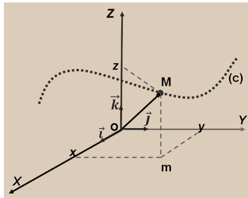
Fig. 16 : Repère cartésiennes dans l'espace
