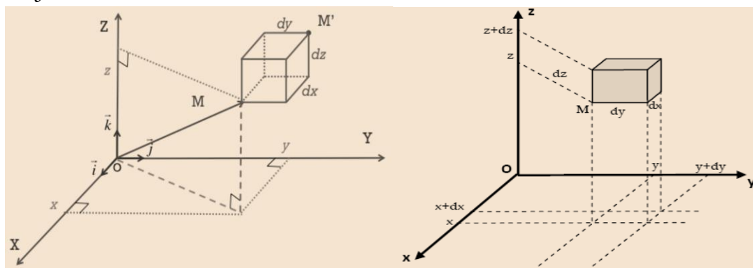
Fig. 18 : représentation de volume élémentaire d^3V = dx \cdot dy \cdot dz
