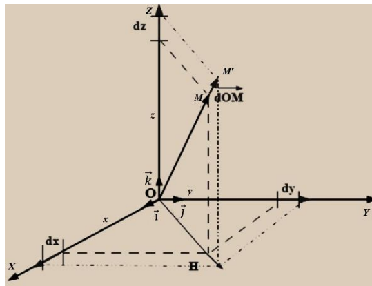
Fig. 17 : Déplacement élémentaire en coordonnées cartésiennes
