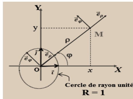
Fig. 18: Les coordonnées polaires (\rho, \phi) et la base associée (\vec{e}_\rho, \vec{e}_\phi)
