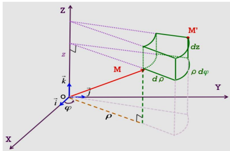
Fig. 22 : Volume élémentaire en coordonnées cylindrique
