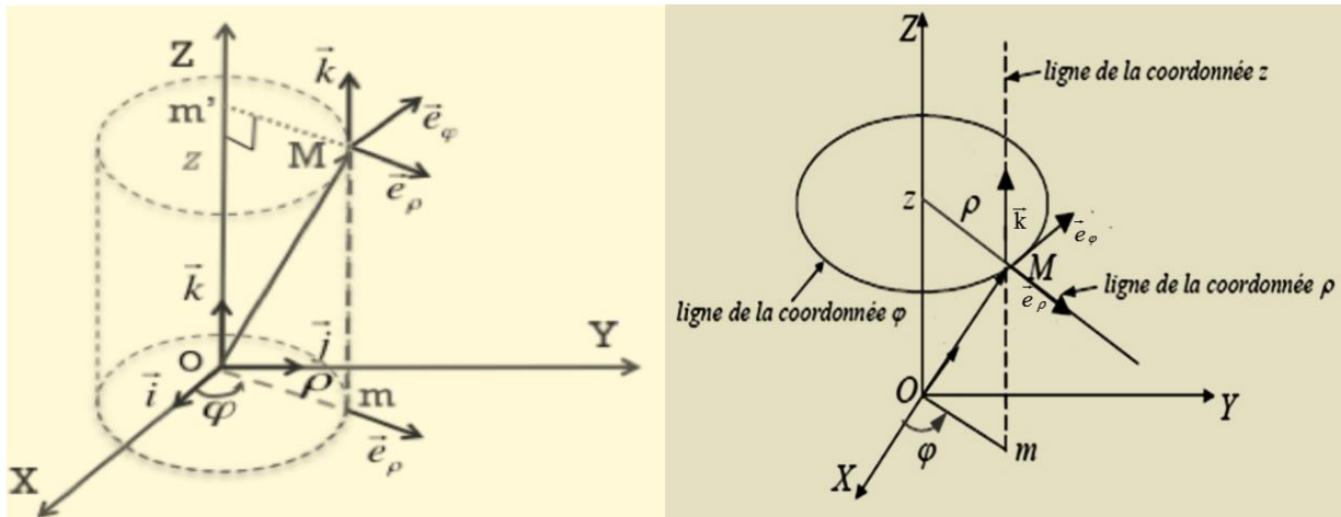
Fig. 20 : Le système de coordonnées cylindriques
